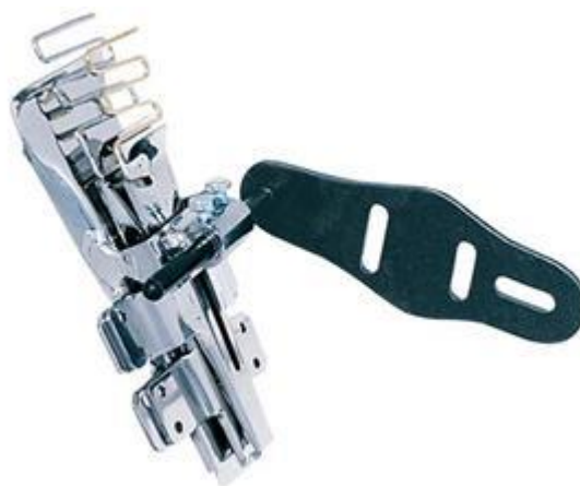
E119 zwijacz do naszywania trzech lampasów do gumiar ki/paskarki. ATTACHMENT FOR THREE RIBBONS BINDED (UP TO UP)
