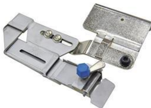
E129B regulowany podajnik do wszywania gumy/taśmy z naprężaczem do overloka. OVERLOCK MACHINE ELASTIC ATTACHMENT FROM SIDE
