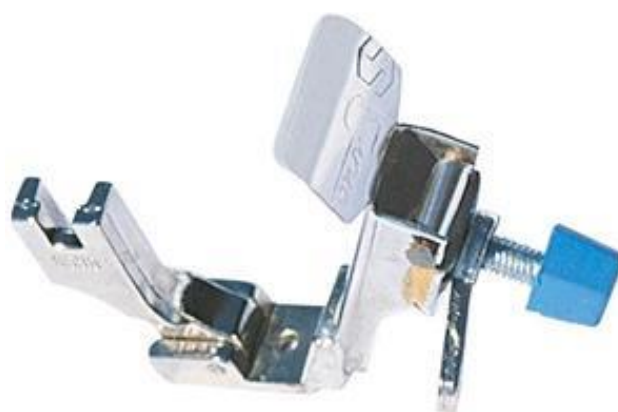
C221 podajnik do gumy z naprężaczem i uchwytem do overloka. UPPER RUBBER ATTACHMENT FOR OVERLOCK MACHINES
