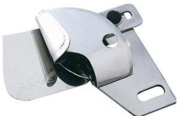
T163 przyrząd do łączenia materiałów do 2-igłówki płaskiej. BOTTOM OPEN DOUBLE NEEDLE SIDE STITCHING ATTACHMENT
